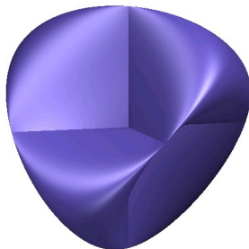
Steinerova ploha
