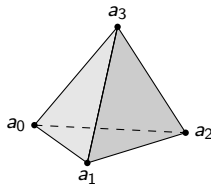
3-simpleks
